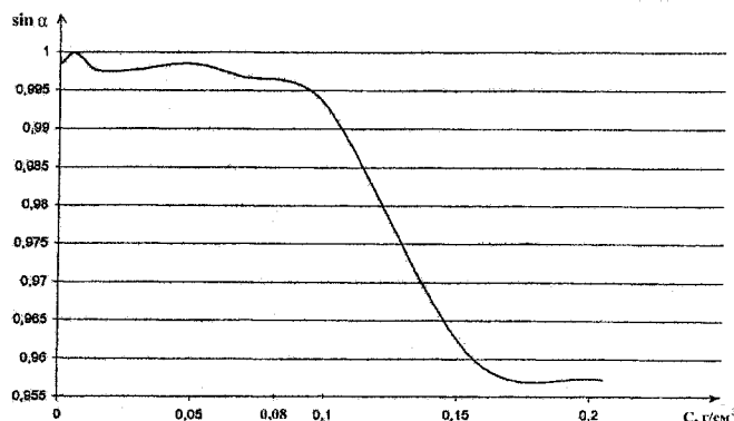
Рис. 4. Зависимость синуса угла между ветвями дендрита от концентрации примесей \text{CuSO}_4
