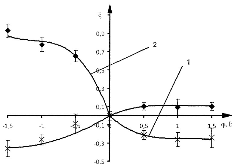
Рис. 3. Зависимость коэффициента чувствительности скорости пластической деформации к изменению внешнего напряжения от потенциала при температуре 296 К (кривая 1), 333 К (кривая 2)
