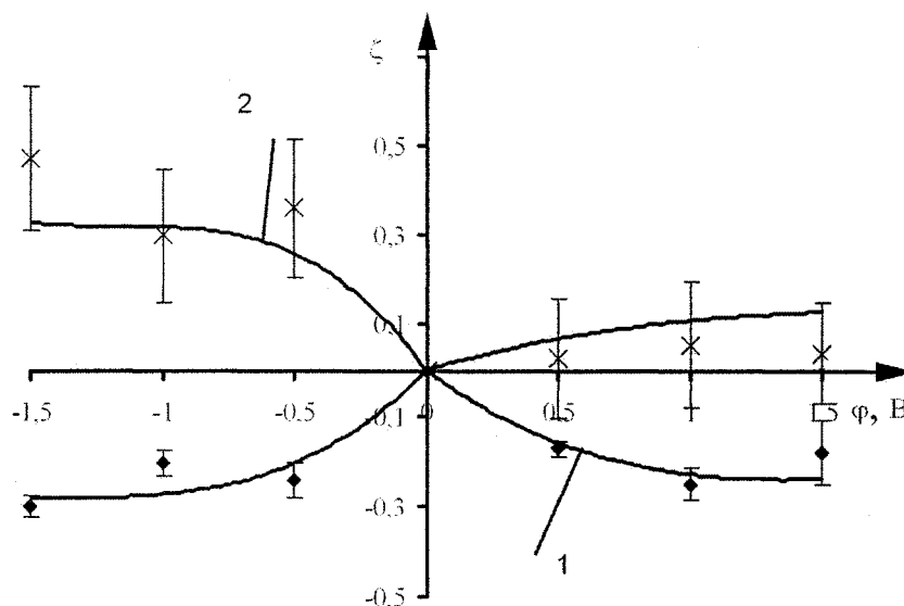
Рис. 2. Зависимость относительного изменения активационного объема от величины электрического потенциала при температуре 296 К (кривая 1), 333 К (кривая 2)
