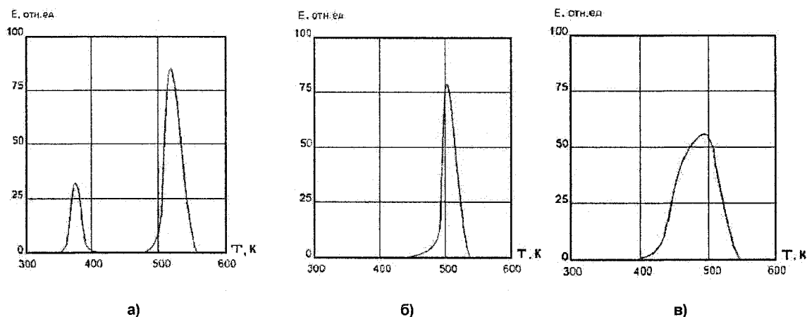
Рис. 5. Зависимость выхода ТЛ трех групп образцов Al_2O_3:Ti^{3+}:Cr^{3+}
