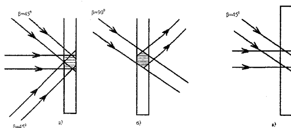
Рис. 3. Голографическая запись в фотопьезоэлектрике: а) запись элементарной голограммы; б) восстановление; в) стирание записи
