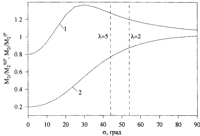
Рис. 2. Зависимости отношений M_{2i}/M_2^{90^\circ} (1) и M_{2i}/M_2^{0^\circ} (2) от дисперсии \sigma
