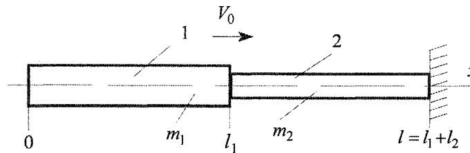
Рис. 1. Схема удара однородных стержней при неударяющих связях
