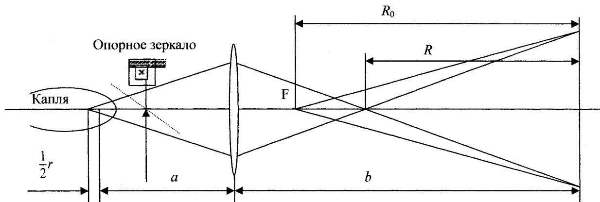
Рис. 7. Определение радиуса кривизны капли интерференционным методом
