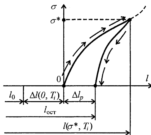
Рис. 3. Остаточное удлинение
