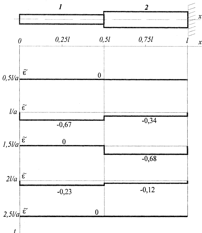
Рис. 5. Диаграмма относительной продольной деформации
