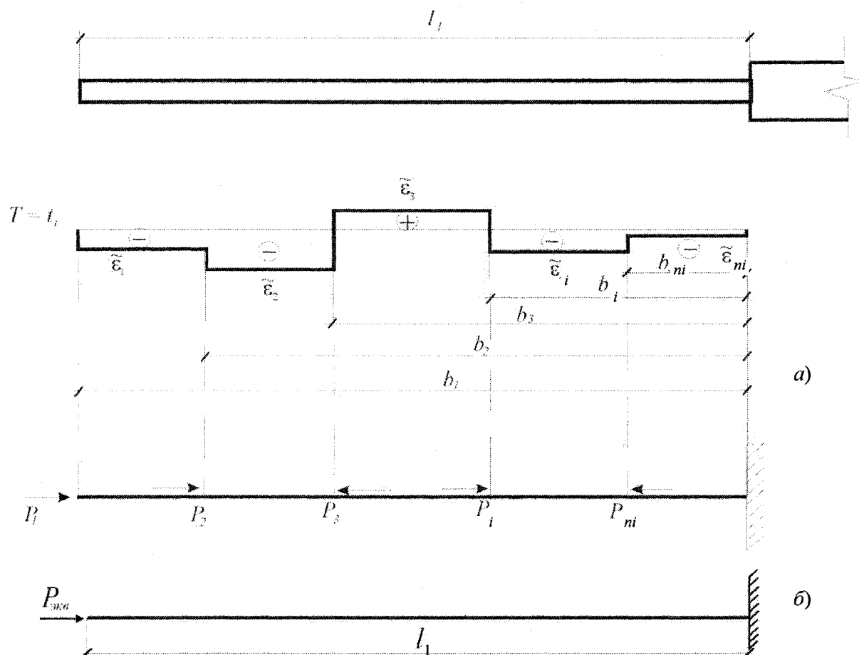
Рис. 2. а) диаграмма относительной продольной деформации для одного из участков произвольной многоступенчатой стержневой системы; б) эквивалентная схема нагружения рассматриваемого однородного участка стержневой системы
