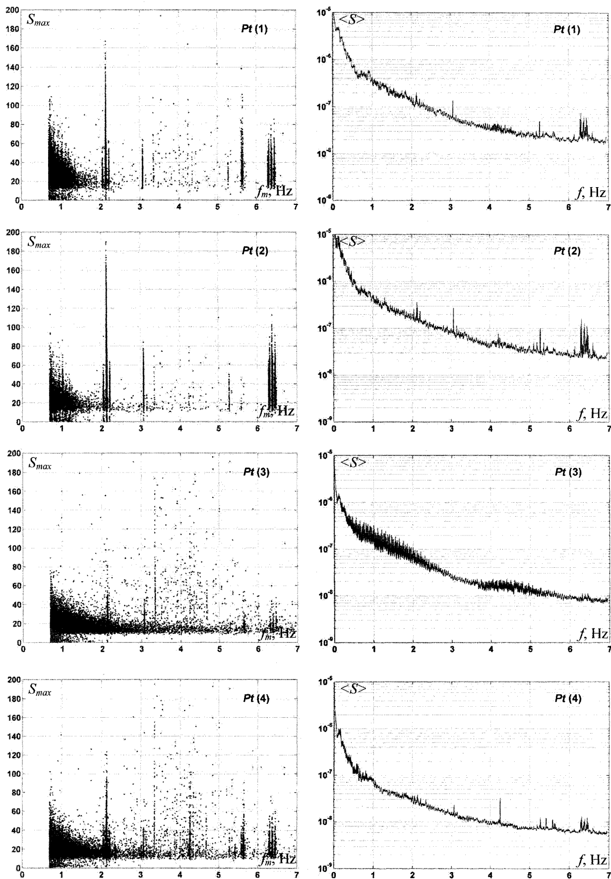
Рис. 2. Кластеры флуктуаций проводимости образцов платины (Pt(1)–Pt(4)) в координатах S_{max} – f_m (слева) и усреднённые спектрограммы (справа)
