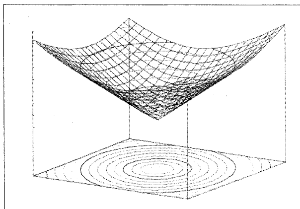
Рис. 5. Вид функции F в малой окрестности экстремума
