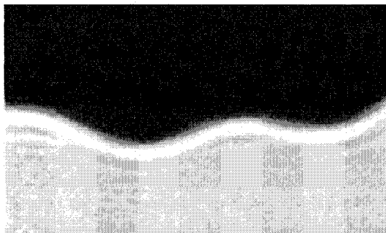
Рис. 1. Волна на поверхности капли, возбужденная сейсмическим шумом
