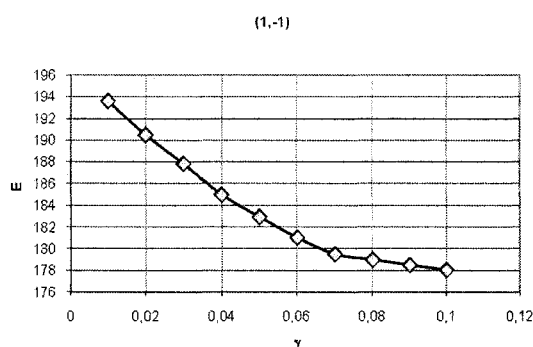
Рис. 10. Зависимость безразмерной энергии топологического солитона (1, -1) от коэффициента диссипации для T7A_1
