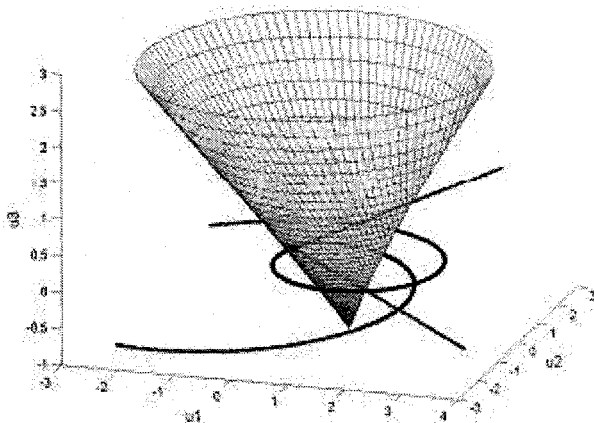
Рис. 2. Конус устойчивости и кривые (4), (13)
