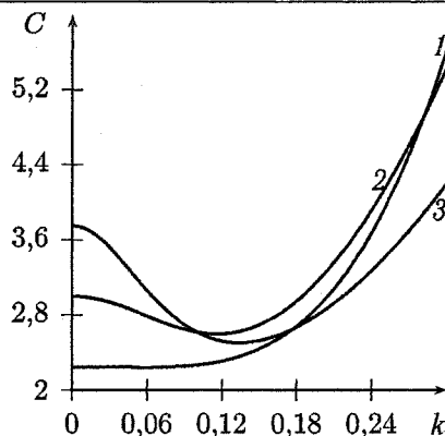
Рис. 2. Фазовые скорости ( Re=10 ): 1 - \tau = -0,15 ; 2 - \tau = 0 ; 3 - \tau = 0,15
