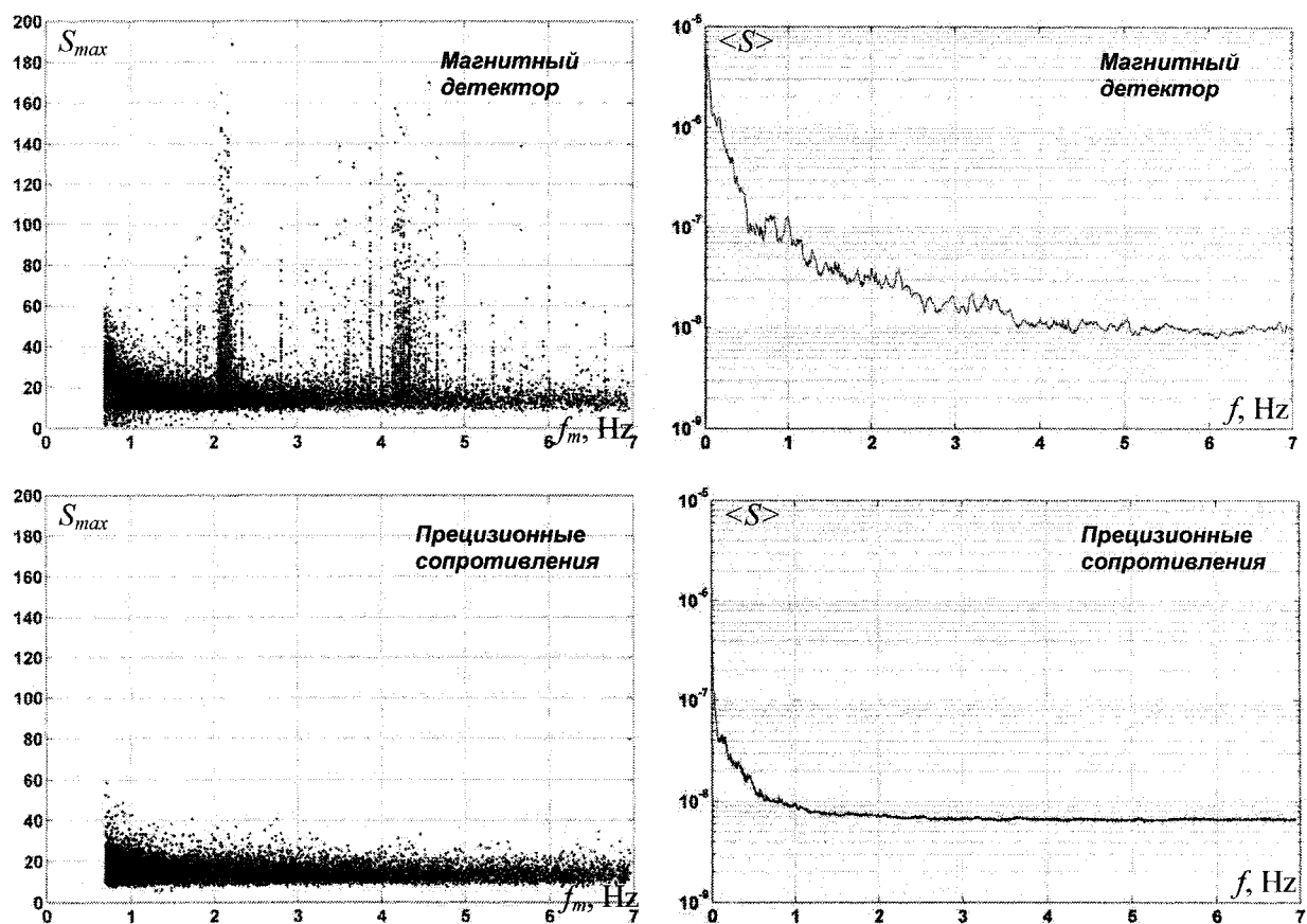
Рис. 3. Кластеры флуктуаций проводимости магнитного детектора и прецизионных сопротивлений в координатах S_{max}-f_m (слева) и усреднённые спектрограммы (справа)
