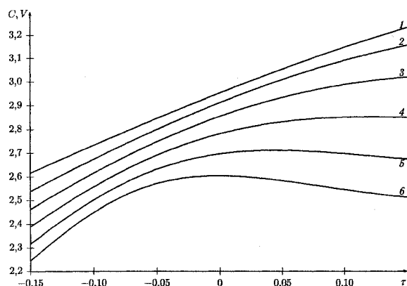
Рис. 6. Фазовые C и групповые V скорости волн максимального роста: 1 – Re = 5 ; 2 – Re = 6 ; 3 – Re = 7 ; 4 – Re = 8 ; 5 – Re = 9 ; 6 – Re = 10
