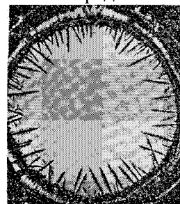
Рис. 2. Начало кристаллизации \text{NH}_4\text{Cl}
