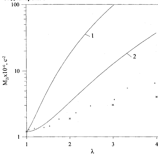
Рис. 3. Зависимость изотропно-порошкового второго момента M_{2i} от степени растяжения \lambda . Точки – экспериментальные значения, найденные в данной работе (•) и в [3] (+). Сплошные линии – теоретические кривые, полученные в предположении гауссовского (1) и ланжевеновского (2) распределений расстояний между узлами химических сшивок и аффинной деформации образца
