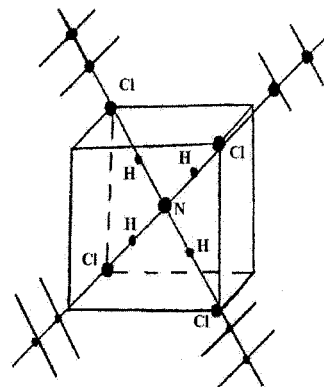
Рис. 3. Элементарная ячейка кристалла \text{NH}_4\text{Cl} кубической симметрии
