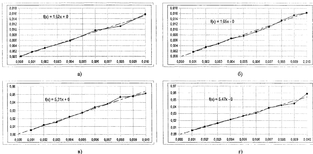
Рис. 6. Зависимости стандартного отклонения коэффициента поверхностного натяжения (мН/м) от стандартного отклонения точек расчетного и экспериментального профилей капли (мм) при различном выборе варьируемых параметров. Функция f(x) – уравнение линейного тренда, показанного пунктиром
