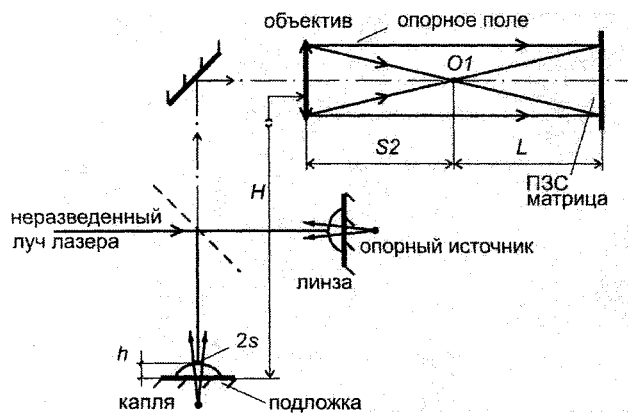
Рис. 1. Схема эксперимента
