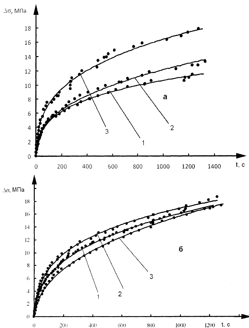
Рис. 1. Изменение глубины релаксации от времени испытания в обычных условиях (кривая 1), при потенциале поверхности -1 В (кривая 2) и +1 В (кривая 3). Температура испытания: а) 296 К, б) 333 К
