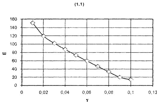
Рис. 6. Зависимость безразмерной энергии топологического солитона (1, 1) от коэффициента диссипации
