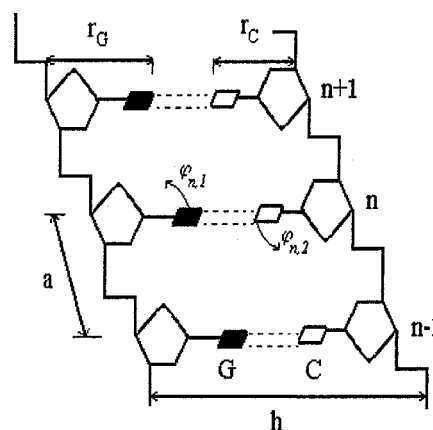
Рис. 1. Фрагмент двойной спирали ДНК, состоящей из трех пар оснований вида GC или (АТ). Расстояние между основаниями вдоль цепи a = 3,4 \text{ \AA} , расстояние между цепями h = 16,15 \text{ \AA} [3, 4]
