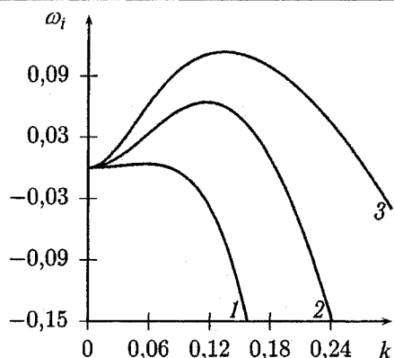
Рис. 1. Инкремент жидкой пленки ( Re = 10 ): 1 - \tau = -0,15 ; 2 - \tau = 0 ; 3 - \tau = 0,15
