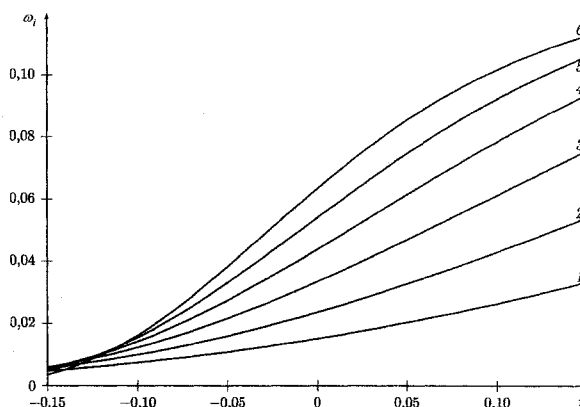
Рис. 7. Инкременты \omega_i волн максимального роста: 1 – Re = 5 ; 2 – Re = 6 ; 3 – Re = 7 ; 4 – Re = 8 ; 5 – Re = 9 ; 6 – Re = 10
