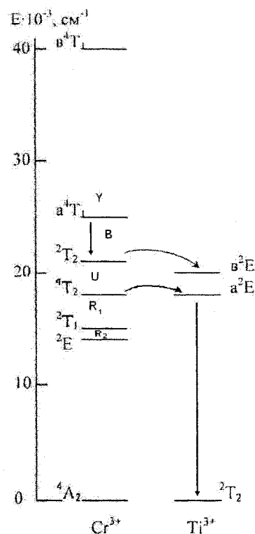
Рис. 4. Энергетические уровни иона титана
