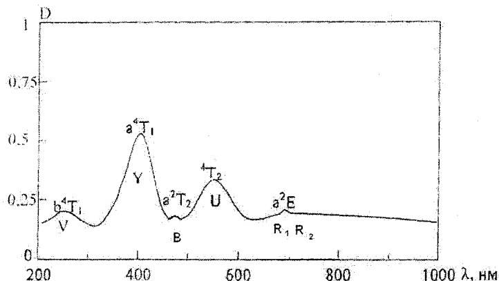
Рис. 1. Кривая спектрального поглощения рубина, содержащего ионы хрома
