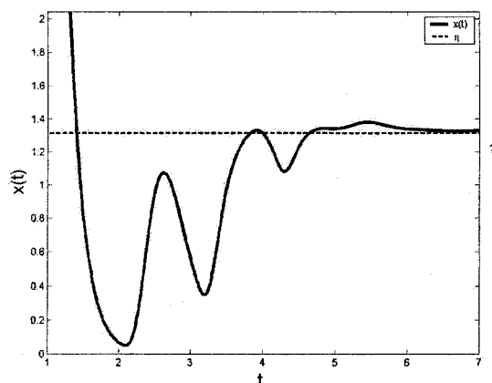
Рис. 1. Отделимость от нуля устойчивого решения модели с параметрами из первой части теоремы 1
