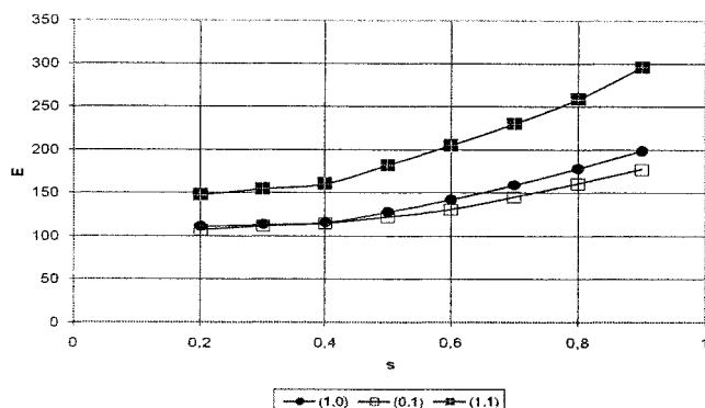
Рис. 8. Зависимости безразмерной энергии солитонов от безразмерной скорости ( s ) для T7A_1
