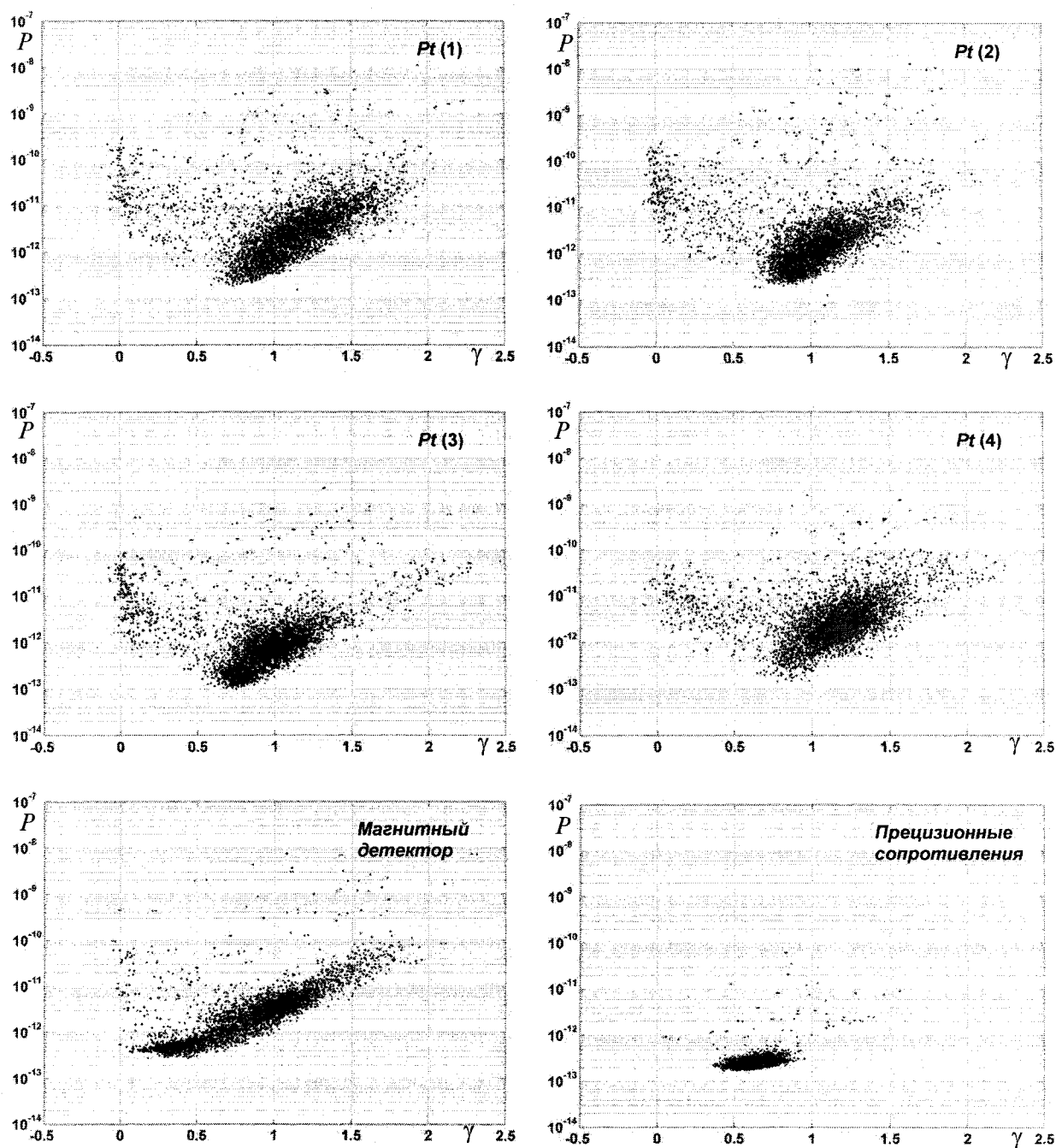
Рис. 1. Кластеры флуктуаций проводимости образцов платины (Pt(1)–Pt(4)), а также магнитного детектора и прецизионных сопротивлений в координатах P – \gamma
