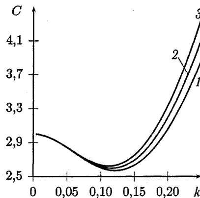
Рис. 4. Фазовые скорости ( Re = 10 ): 1 - \Delta\sigma = -10\% ; 2 - \Delta\sigma = 0 ; 3 - \Delta\sigma = 10\%
