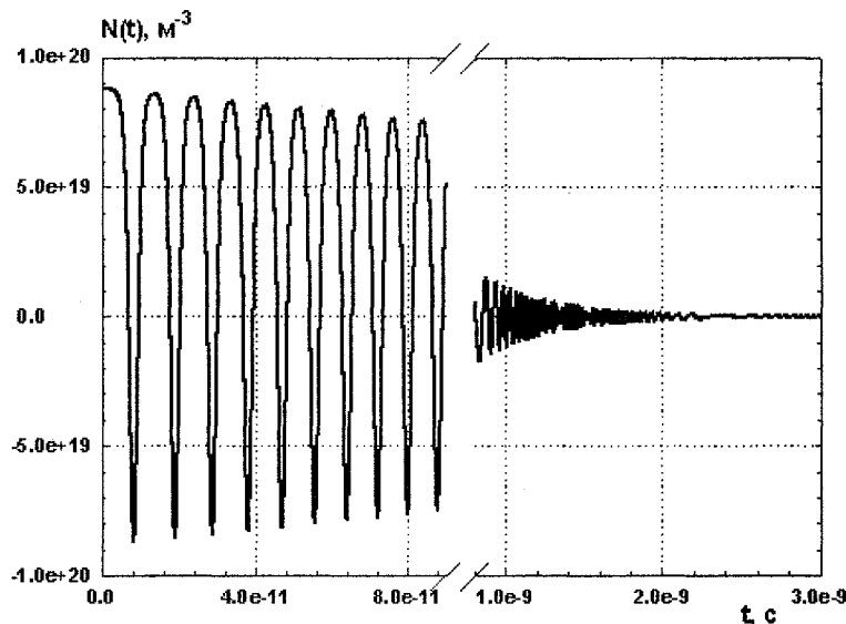
Рис. 3. Зависимость населенности от времени
