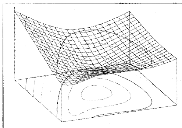
Рис. 4. Вид целевой функции F в области экстремума. Использована специальная система координат, оси которой совпадают с полуосями одного из эллипсов
