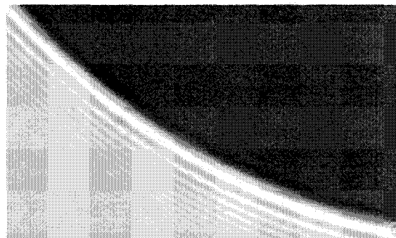
Рис. 2. Дифракционная картина у поверхности капли
