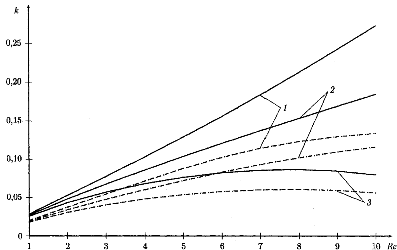
Рис. 5. Области неустойчивости жидкой пленки: 1 – режим противотока ( \tau = 0,15 ); 2 – \tau = 0 ; 3 – режим прямотока ( \tau = -0,15 ); сплошные линии – кривые нейтральной устойчивости; пунктирные линии – кривые максимального роста
