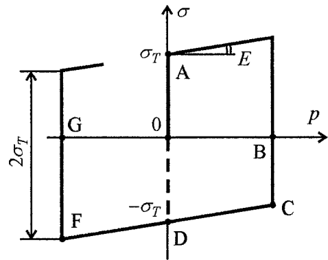
Рис. 4. Модель Ишлинского–Прагера
