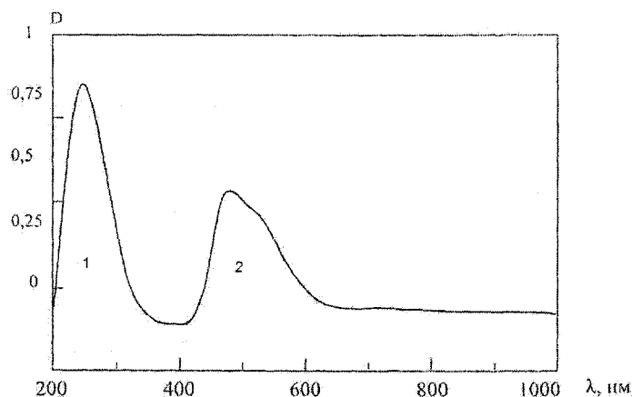
Рис. 2. Кривая спектрального поглощения рубина, содержащего ионы хрома и титана
