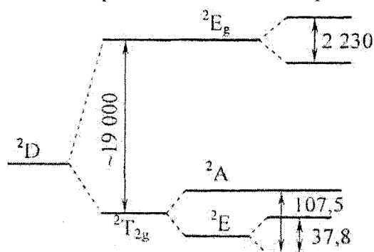
Рис. 3. Электронная конфигурация 3d^1 иона титана
