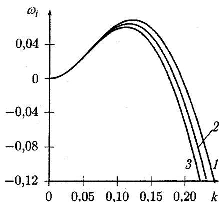
Рис. 3. Инкремент жидкой пленки ( Re = 10 ): 1 - \Delta\sigma = -10\% ; 2 - \Delta\sigma = 0 ; 3 - \Delta\sigma = 10\%
