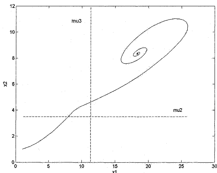
Рис. 3. Отделённость от нуля устойчивого решения модели с параметрами из п. 4 теоремы 2
