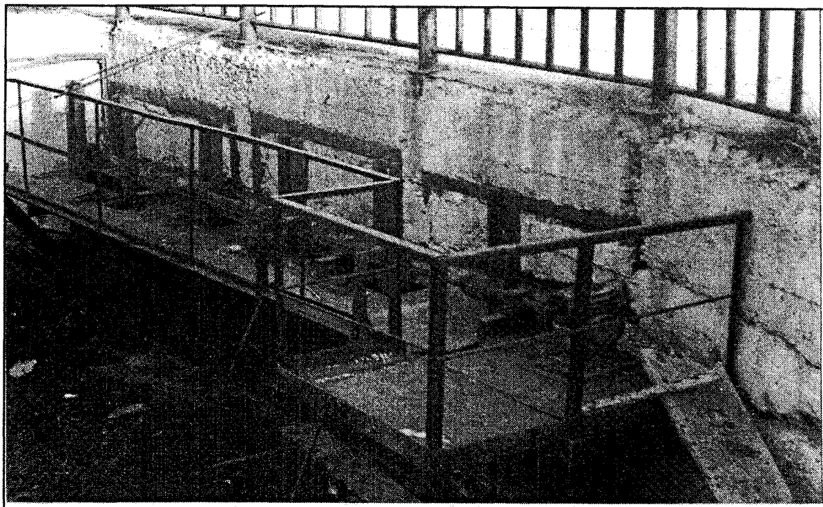
Рис. 1 Современное механическое устройство для подъема ставней со стороны пруда
