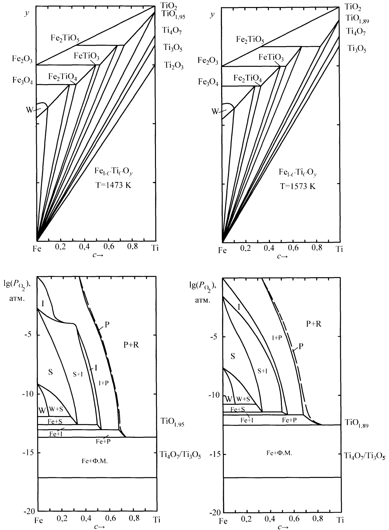
Рис. 5. Изотермические сечения диаграммы состояния системы Fe-Ti-O при температуре 1473 и 1573 K W – твердый раствор титана в вюстите, S – твердый раствор магнетита и ульвошпинели, I – твердый раствор гематита и ильменита, P – ферропсевдобрукит, R – рутил, Ф.М. – фазы Магнели
