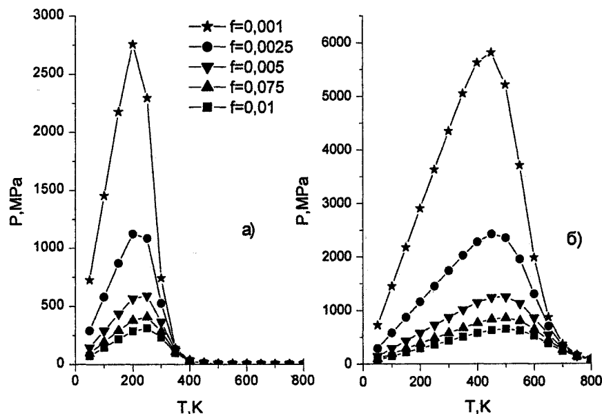
Рис. 4. Зависимость давления водорода в порах от температуры и доли пор при различных значениях энергии активации растворения водорода: E = 17\ 185 Дж/моль (а) и E = 37\ 185 Дж/моль (б). Данные для промежуточного значения E = 27\ 185 Дж/моль приведены на рис.16
