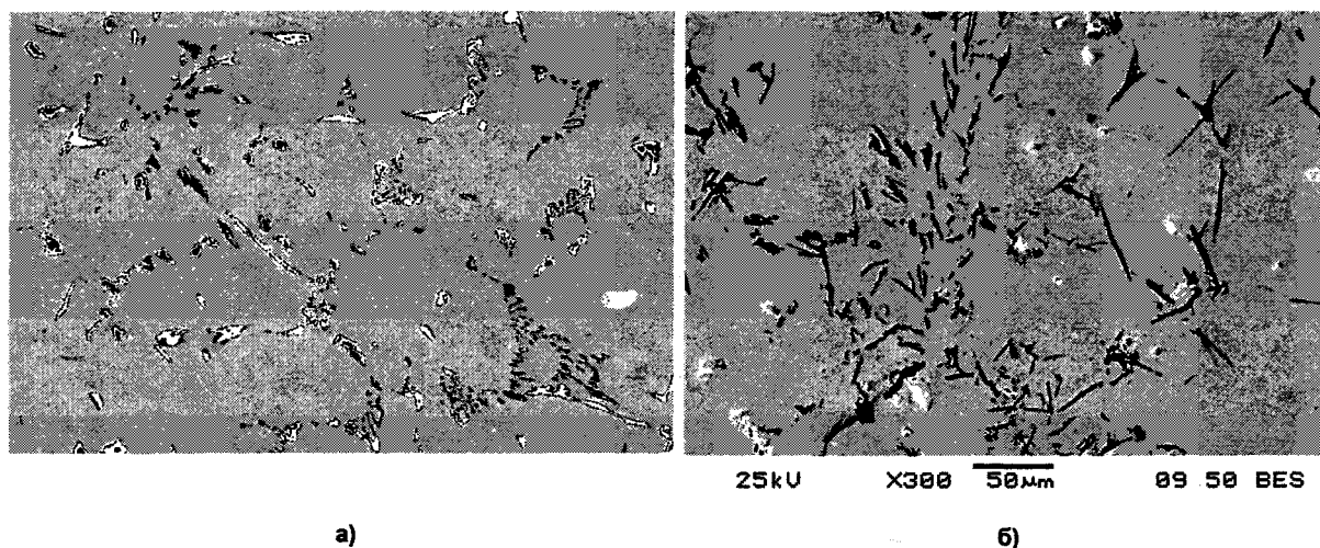
Рис. 4. Микроструктуры необлученного (а) и облученного (б) образцов соответственно после закалки и длительного старения при 190 °С, X300
