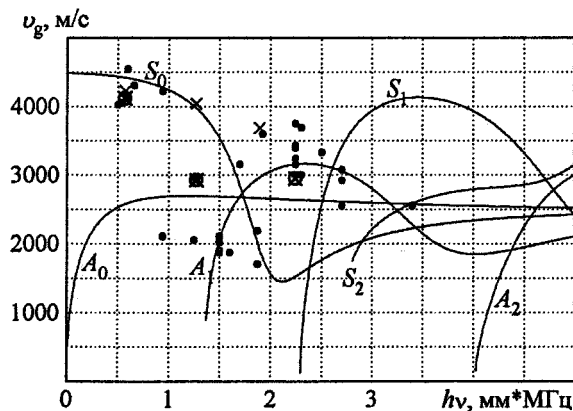
Рис. 5. Зависимость групповой скорости нормальных волн \nu_g от параметра \nu h -- расчет, эксперимент: • – ПП, ⊗ – КПВТП, × – ЭМАП. d = 4,00 мм, q = 2,30 МВт/см 2
