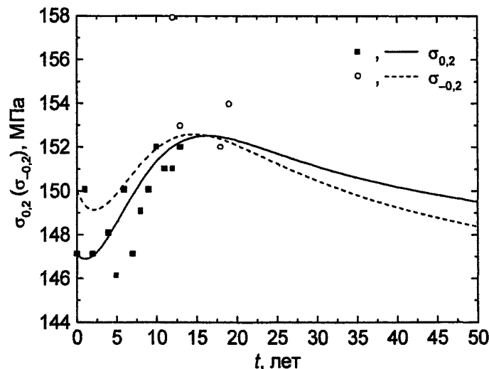
Результаты расчёта изменения пределов текучести при растяжении и сжатии в зависимости от времени выдержки при 20 °С. Точки — экспериментальные данные
