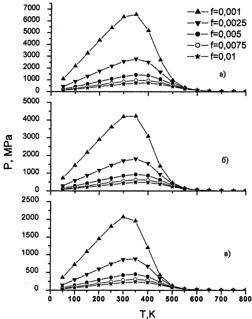
Рис. 1. Влияние температуры и объемной доли пор f на давление водорода для различного содержания водорода в железе: а – 2,5; б – 5; в – 7,5 см 3 /г
