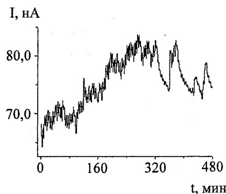
Рис. 1. Кинетика тока гелевой системы оксигидрата циркония
