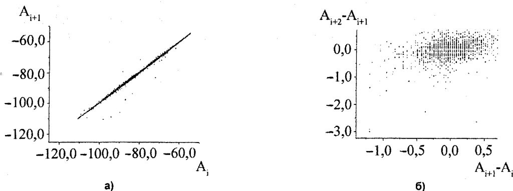
Рис. 4. Линейные участки, окруженные стохастическим слоем. Отображения первого (а) и второго (б) возвращения. Образцы синтезированы при pH = 9,25, n_{ZrO_2} = 0,0094 моль; возраст геля 10 суток
