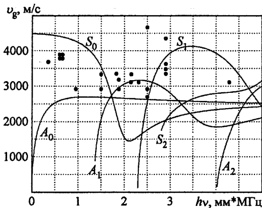
Рис. 3. Зависимость групповой скорости нормальных волн \nu_g от параметра \nu h -- расчет, • – эксперимент d = 2,00 мм, q = 50,0 МВт/см 2
