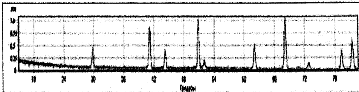
Рис. 3. Фрагмент рентгенограммы образца корунда, полученного термообработкой в замкнутом объеме фракции гиббсита 100–140 мкм. Излучение – Co K α
