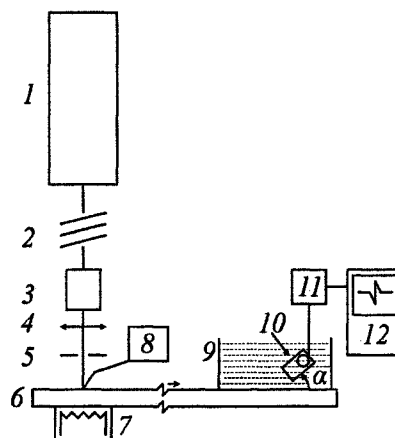
Рис. 1. Схема экспериментальной установки: 1 – лазер, 2 – оптический attenuатор, 3 – измеритель мощности лазерного излучения, 4 – линза, 5 – диафрагма, 6 – ферромагнитная пластина, 7 – нагреватель, 8 – измеритель температуры, 9 – ванна с водой, 10 – прямой пьезоискатель продольных волн и устройство для его закрепления и поворота, 11 – усилитель, 12 – осциллограф
