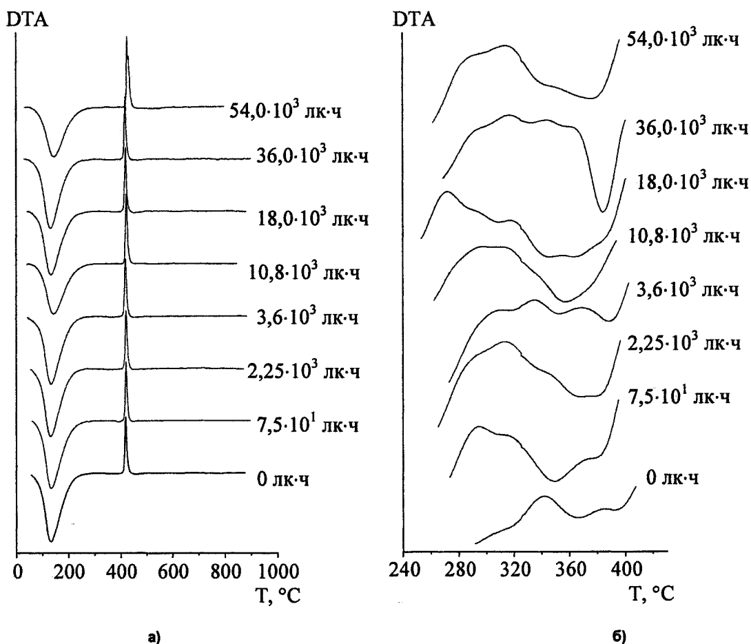
Рис. 2. Изменение профиля кривых ДТА (а) и второго эндоэффекта (б) при возрастании дозы облучения ультрафиолетом
