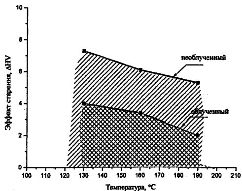
Рис. 2. Зависимость эффекта старения сплава Al-4%Cu от температуры старения
