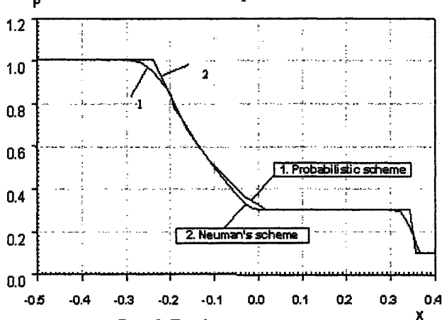
Рис. 2. Профиль давления
