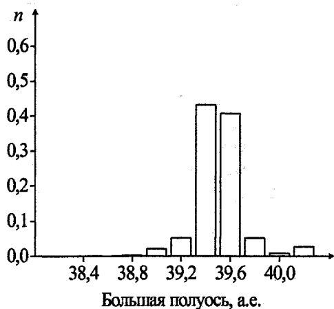
Рис. 1. Распределение больших полуосей объектов резонанса 2/3 в момент окончания миграции Нептуна
