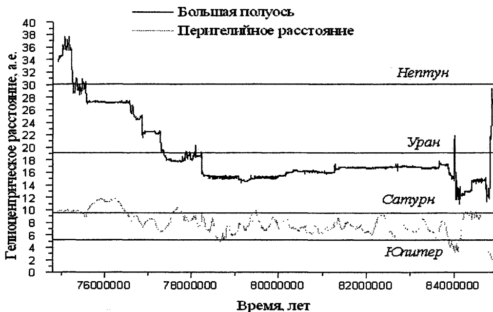
Рис. 1. Динамическая эволюция элементов орбит объекта I, испытавшего a -захват
