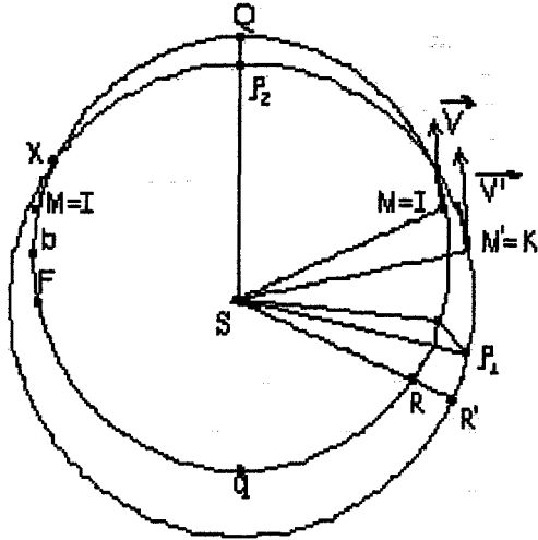
Рис. 1. Орбита кометы A_2 с наибольшим афелийным расстоянием
