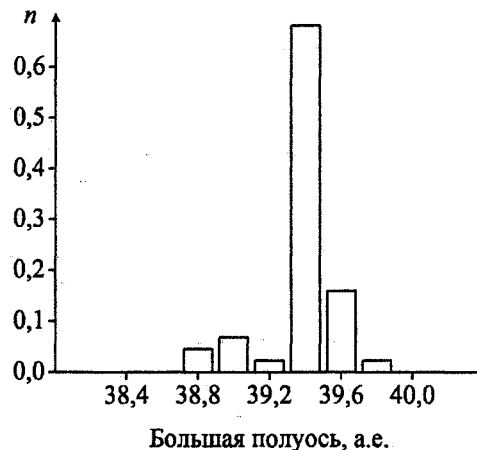
Рис. 2. Распределение больших полуосей объектов резонанса 2/3 после долговременной эволюции
