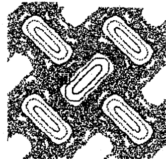
Рис. 6. Стохастическая паутина Детали фазового портрета отоб- ражения \tilde{M}_4 : часть паутины при K_0 = 2 , размер квадрата 4\pi \times 4\pi (а) [4]
