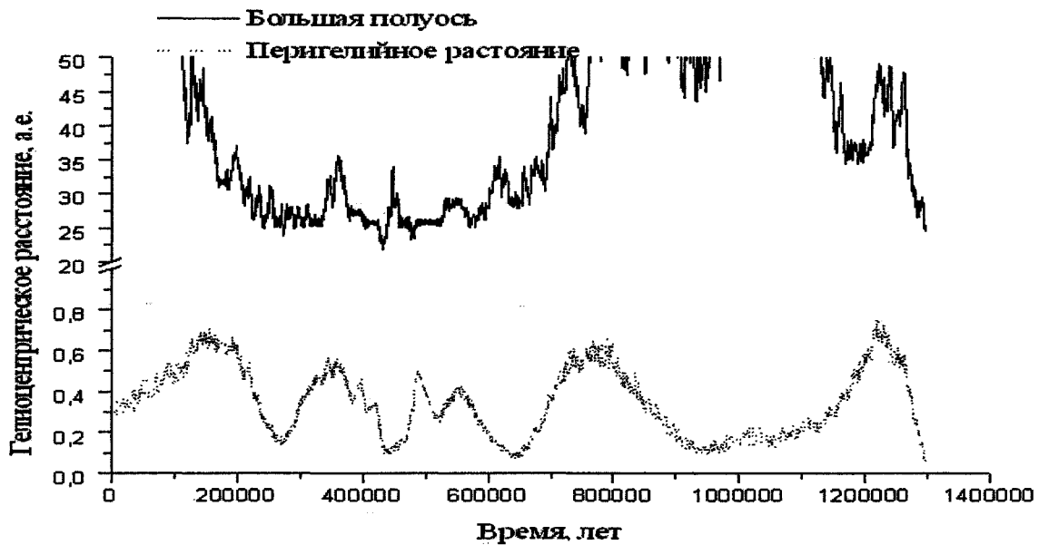
Рис. 3. Динамическая эволюция элементов орбит объекта III, испытавшего q-захват
