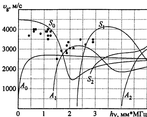
Рис. 4. Зависимость групповой скорости нормальных волн \nu_g от параметра \nu h -- расчет, • – эксперимент d = 3,00 мм, q = 20,0 МВт/см 2
