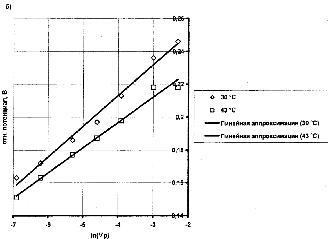
Рис. 3. Зависимость отн. потенциала анодного мах от корня квадратного из скорости развертки (а), либо от натурального логарифма скорости развертки потенциала(б) в температурном ряду 22...43 °С
