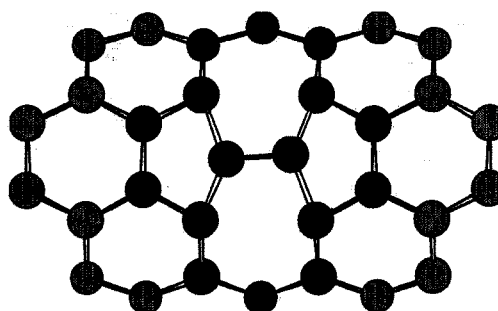
Рис. 5. Фрагмент поверхности нанотрубки, содержащей дефект переключения связей 5-7-7-5
