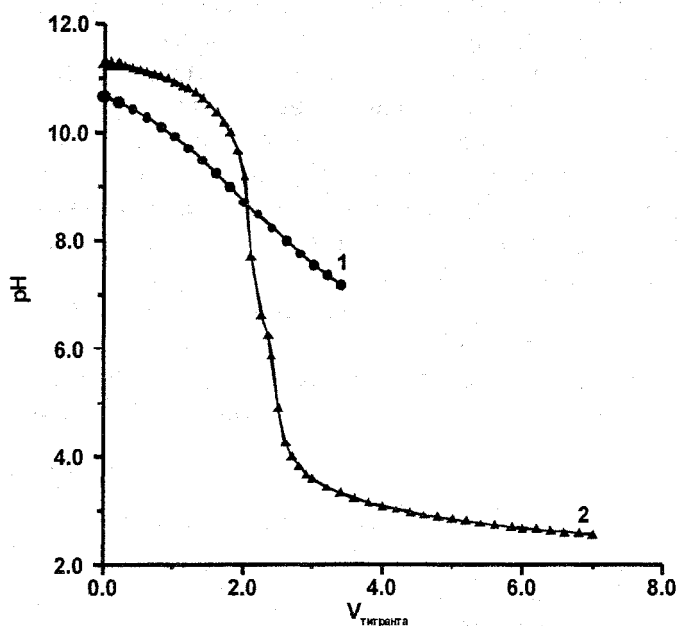
Рис. 2. Пример кривой титрования Fe-геля с сорбированным фосфат-ионом, состаренного в 1,0 M NaCl, среда 0,5 M NaCl: 1 – кривая титрования Fe-геля; 2 – «холостой» опыт
