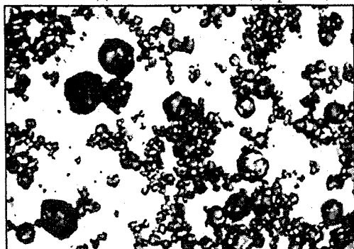
Рис. 1. Микрофотография образца исходного гиббсита, масштаб: 1 см – 150 мкм
