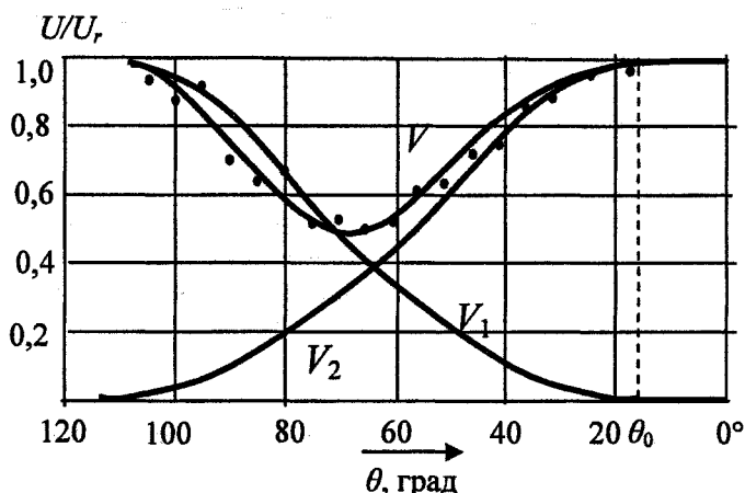
Рис. 5. Зависимости коэффициентов прохождения волн на плоскость от угла \theta
