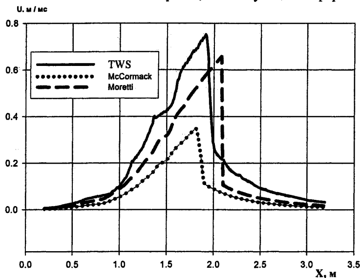
Рис. 5. Распределение скорости по длине сопла
