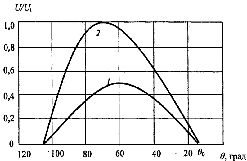
Рис. 2. Распределение амплитуд смещений в объемных волнах в зависимости от угла клина. 1 – продольные волны, 2 – сдвиговые волны
