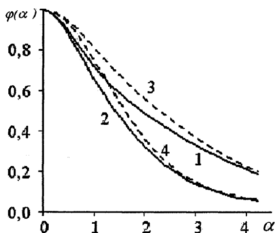
Влияние магнитного поля на плотность массового потока к поверхности диска: 1 – \sigma = 1,0 ; Pr = 10^3 , 2 – \sigma = 1,0 ; Pr = 10^2 , 3 – \sigma = 0,1 ; Pr = 10^3 , 4 – \sigma = 0,1 ; Pr = 10^2
