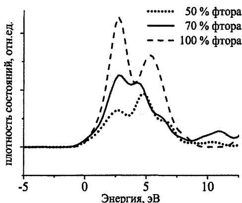
Рис. 1. Модификация плотности свободных состояний атомов фтора по мере карбонизации ПВДФ
