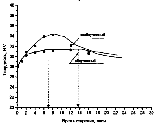
Рис. 1. Изменение твердости сплава Al-4 % Cu в процессе старения: а – при 100 °С, б – при 130 °С, в – при 160 °С
