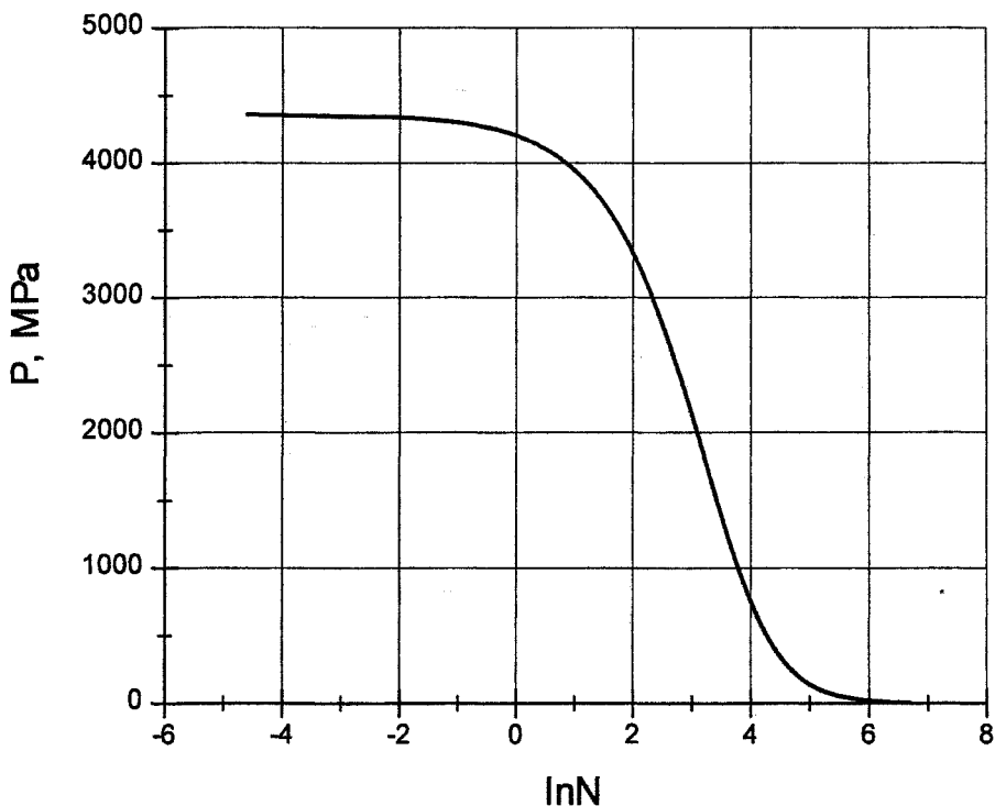
Рис. 5. Влияние растворимости водорода в железе на давление водорода в порах: N = \Lambda_1 / \Lambda_1(\text{Fe}) , где \Lambda_1(\text{Fe}) = 8,78 \cdot 10^{-4} \text{ см}^3/100 \text{ г} – коэффициент растворимости водорода в железе, а \Lambda_1 – различные возможные значения данного коэффициента для сплавов железа
