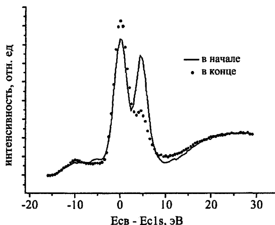
Рис. 4. Модификация спектров остовного уровня атомов углерода ПВДФ в процессе радиационной карбонизации
