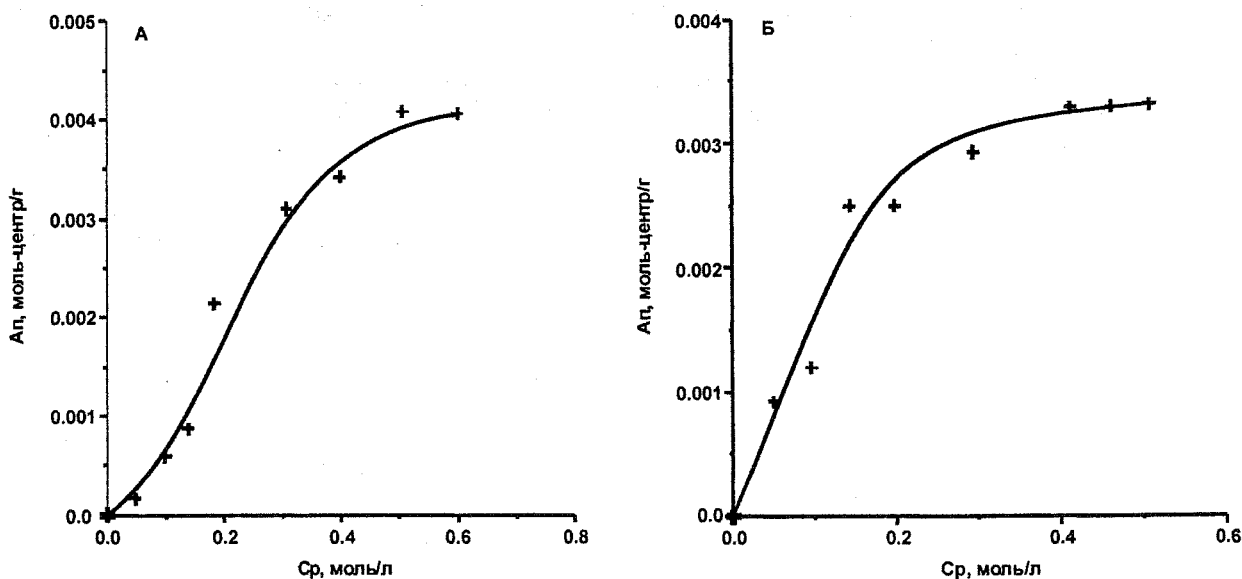
Изотермы адсорбции CO_3^{2-} -ионов из водных растворов Na_2CO_3 на оксигидроксидах железа(III) (А) и алюминия (Б) с pH осаждения 9
