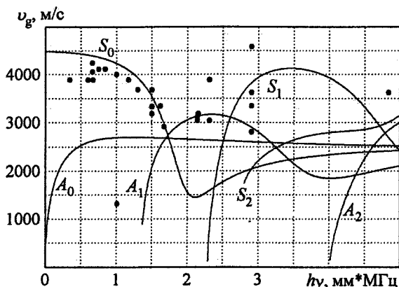
Рис. 2. Зависимость групповой скорости нормальных волн \nu_g от параметра \nu h -- расчет, • – эксперимент d = 1,00 мм, q = 180 МВт/см 2
