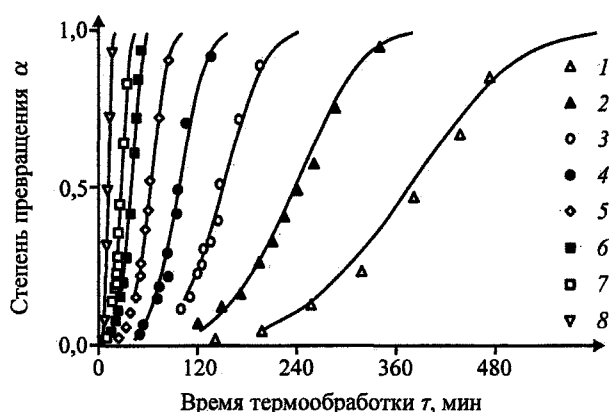
Кинетические кривые фазового превращения гиббсит → бемит: температуры термообработки 1 – 180, 2 – 185, 3 – 190, 4 – 192, 5 – 195, 6 – 200, 7 – 205, 8 – 210 °C
