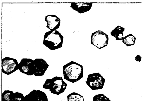
Рис. 4. Микрофотография кристаллов корунда, полученного термообработкой образца фракции гиббсита 100–140 мкм. Масштаб: 1 см – 50 мкм
