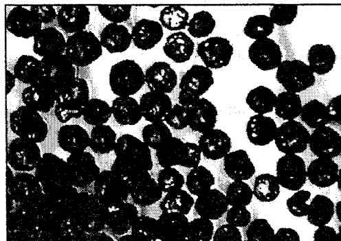
Рис. 2. Микрофотография образца фракции гиббсита 100–140 мкм, масштаб: 1 см – 150 мкм
