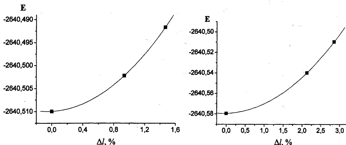
Рис. 7. Зависимость полной энергии от относительного удлинения для нанотрубки (5.0) с расположением дефекта поперек (слева) и вдоль (справа) оси нанотрубки
