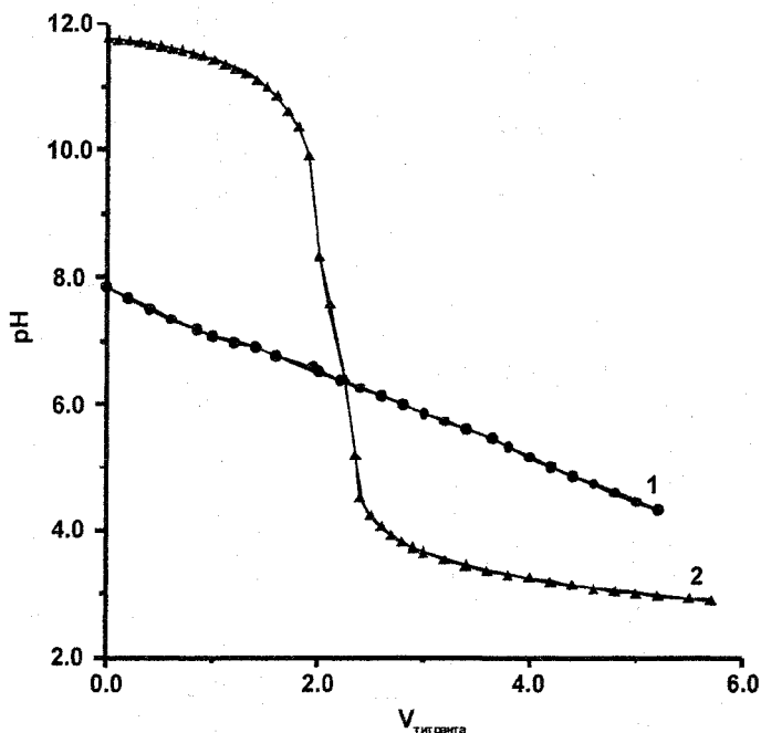
Рис. 3. Пример кривой титрования Zr-геля с сорбированным арсенат-ионом, состаренного в 1,0 M NaCl, среда 0,5 M NaCl: 1 – кривая титрования Zr-геля; 2 – «холостой» опыт
