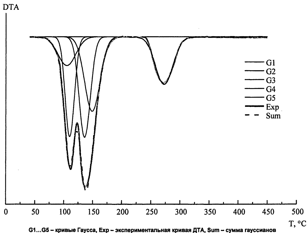
Рис. 1. Аппроксимация экспериментальной кривой ДТА дегидратации сульфата меди ( \text{CuSO}_4 \cdot 5\text{H}_2\text{O} ) функциями Гаусса
