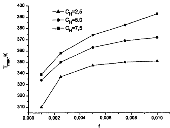
Рис. 2. Влияние концентрации водорода в железе и доли пор f на температуру T_m , при которой давление водорода максимально
