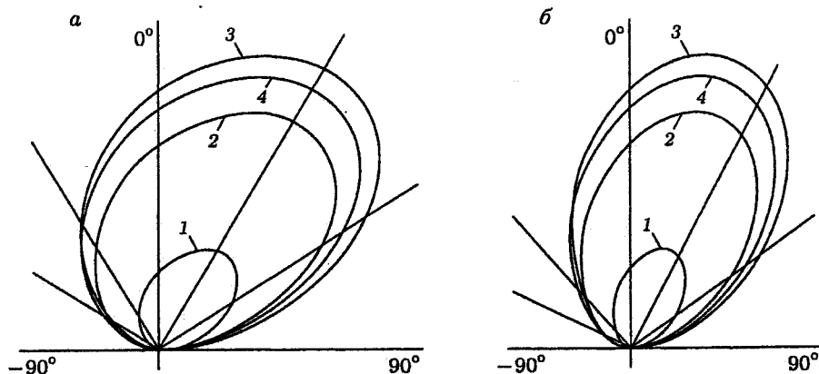
Рис. 3. Диаграмма направленности продольных (а) и сдвиговых (б) волн при различных углах клина. 1 – 150^\circ , 2 – 140^\circ , 3 – 120^\circ , 4 – 100^\circ
