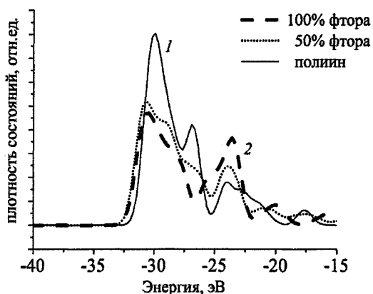
Рис. 3. Плотность состояний остовного уровня атомов углерода ПВДФ, полиина и промежуточного соединения
