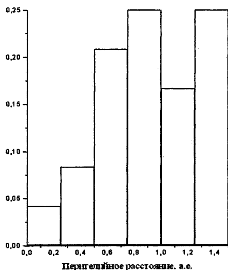
Рис. 1. Наблюдаемое распределение перигелийных расстояний КГТ
