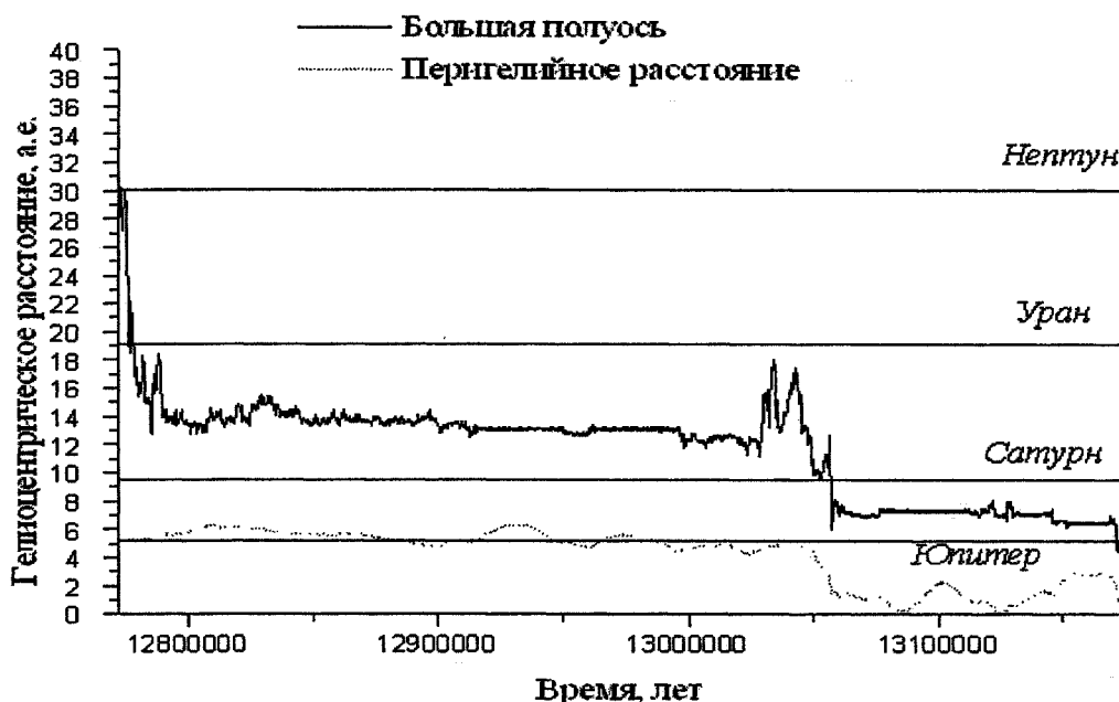
Рис. 2. Динамическая эволюция элементов орбит объекта II, испытавшего \alpha -захват
