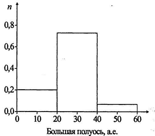
Рис. 5. Распределение наблюдаемых кентавров по большим полуосям
