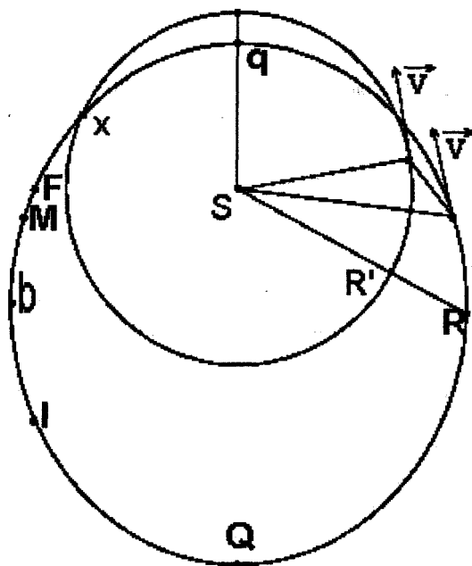
Рис. 3. Наибольшая орбита кометы P 4
