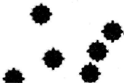
Рис. 5. Геометрия точечных множеств токовых выплесков
