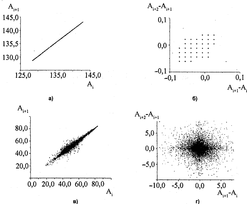
Рис. 2. Регулярный (а, б) и хаотический (в, г) характер отображений. Отображения первого (а, в) и второго возвращения (б, г). Образцы синтезированы при pH = 9,25 , n_{ZrO_2} = 0,0094 моль. Возраст геля 35 суток (а, б), 42 суток (в, г)
