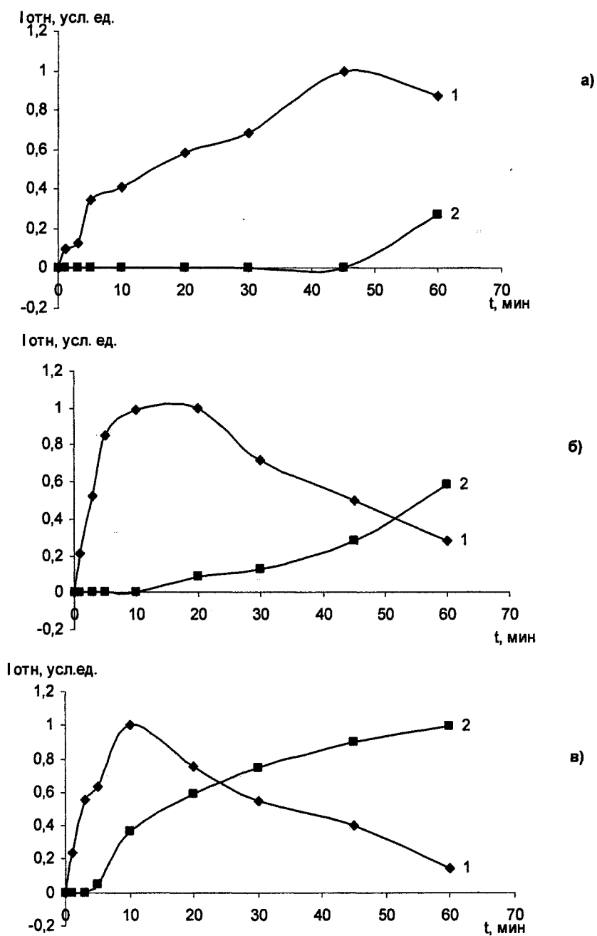
Рис. 1. Фазовый переход анатаза в рутил без добавок \text{Cr}_2\text{O}_3 при различных температурах изотермической выдержки: а) 850 °C; б) 900 °C; в) 1000 °C. 1 – интегральной интенсивности анатаза; 2 – интегральной интенсивности рутила
