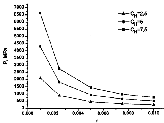
Рис. 3. Зависимость величины максимального давления в порах от концентрации водорода и степени пористости f
