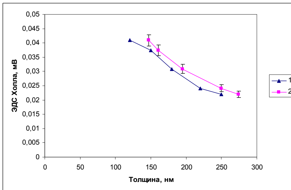
Рис. 2. Зависимость ЭДС Холла от толщины образцов 1 – график от измеренной толщины, 2 – график от рассчитанной толщины по МСЭ
