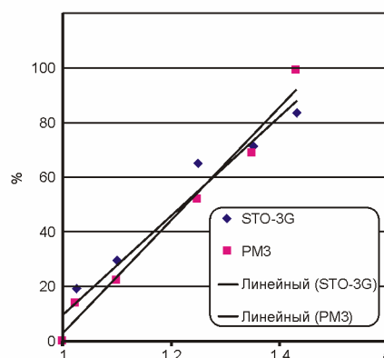
Рис. 6. Зависимость относительного числа комплексов с двумя атомами фосфора, содержащими фтор, от R
