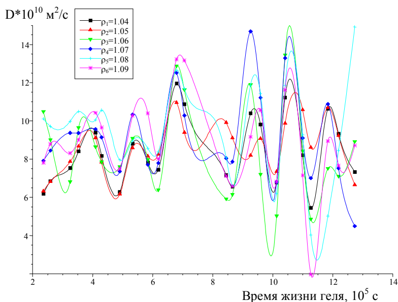
Рис. 1. Диффузия ионов Y3+ в гель кремниевой кислоты при pH = 4.0 ( \rho – плотность исходного раствора метасиликата натрия в г/см^3 )
