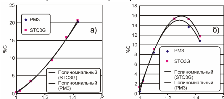
Рис. 3. Относительное число атомов кислорода в комплексе с: а) n = 1 и б) n = 7 в моделях с наборами энергий, полученных полупирическим методом PM-3 и неэмпирическим расчетом с базисом STO-3G
