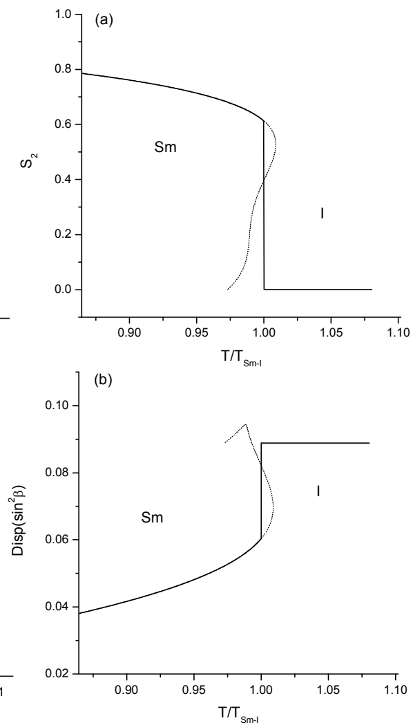
Рис. 5. Нематический порядок (a) и дисперсия межмолекулярных направлений (b) при J_{220} = J_{022} = 0,9J_{202} , J_{222} = -0,9J_{202} , J_{242} = -2,8J_{202}
