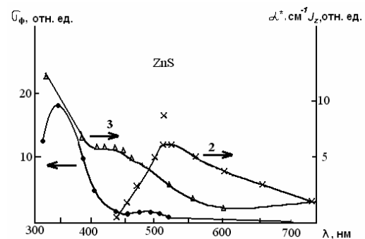
Рис. 2. Спектральное распределение фотовольтаического тока J_z (2), фотопроводимости \sigma_{\phi} (1) и оптического поглощения \alpha^* (3) при T = 143\text{ K} . \beta = 45^\circ
