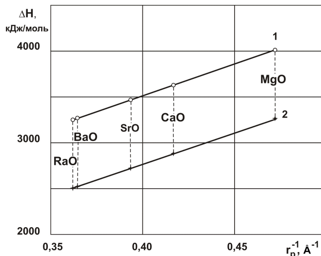
Зависимость энтальпии разрушения кристаллической решетки (1) и энтальпии взаимодействия (2) оксидов ЩЗМ и магния от обратной величины межструктурного расстояния: о – справочные данные, — – результаты расчета
