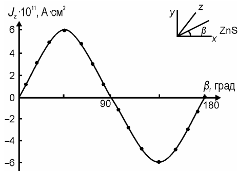
Рис. 1. Ориентационная зависимость плотности фотовольтаического тока J_z в направлении [001]. ( T = 143\text{ K} , I = 2,3 \cdot 10^{-3}\text{ Вт}\cdot\text{см}^{-2} , \lambda = 500\text{ нм} )
