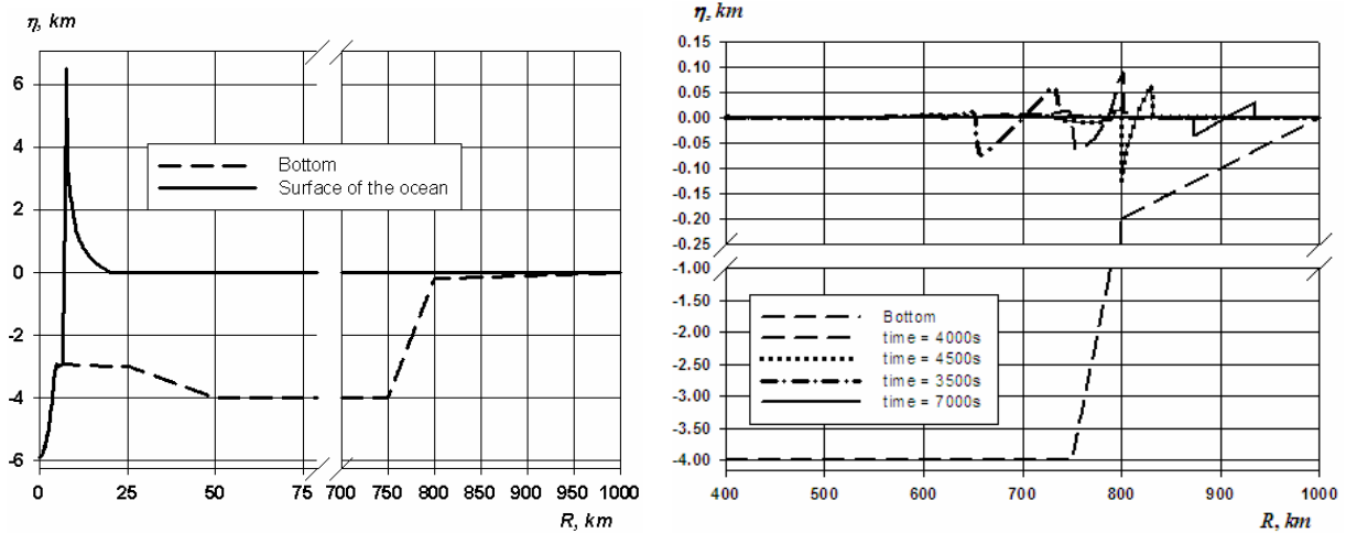
Рис. 4. Профили поверхности воды и дна океана на момент 12 с, полученные из расчетов по коду МЕЧ, и по коду ТМВ на различные моменты времени: 3500 с, 4000 с, 4500 с, 7000 с
