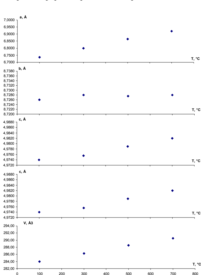
Рис. 2. Политермы параметров элементарной ячейки \beta\text{-Mn}_2\text{V}_2\text{O}_7
