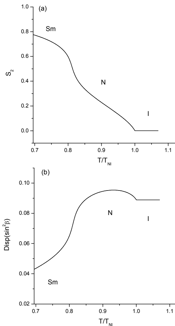
Рис. 4. Нематический порядок (a) и дисперсия межмолекулярных направлений (b) при J_{220} = J_{022} = 0,9J_{202} , J_{222} = J_{242} = -2J_{202}
