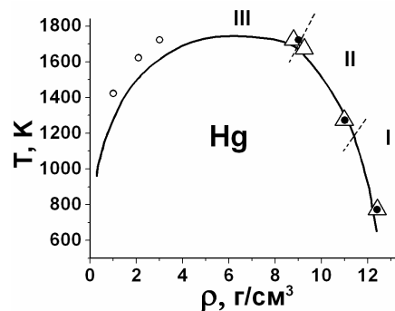
Рис. 2 Фазовая диаграмма ртути: △ – исследуемые модели, ○ – состояния, в которых исследовалась дисперсия звука [3], ● – аномальная дисперсия звука
