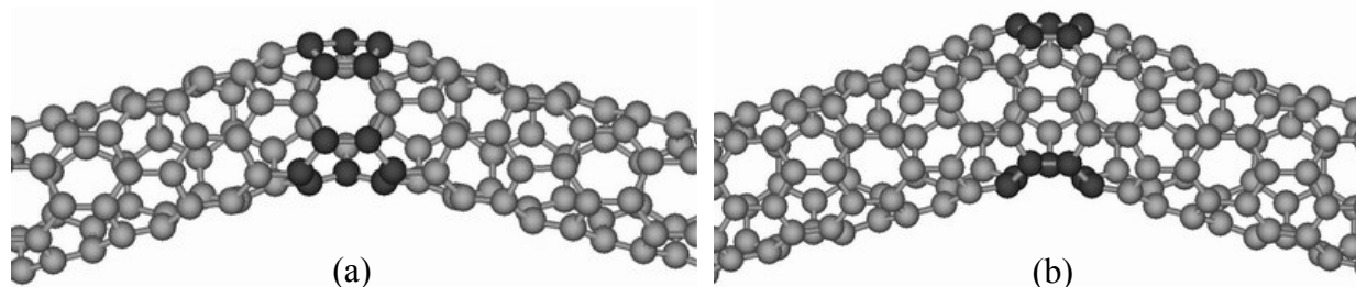
Рис. 4. Структура chiral-chiral соединений пар одинаковых однослойных УНТ: (а) (4,2)–(4,2); (б) (5,2)–(5,2)
