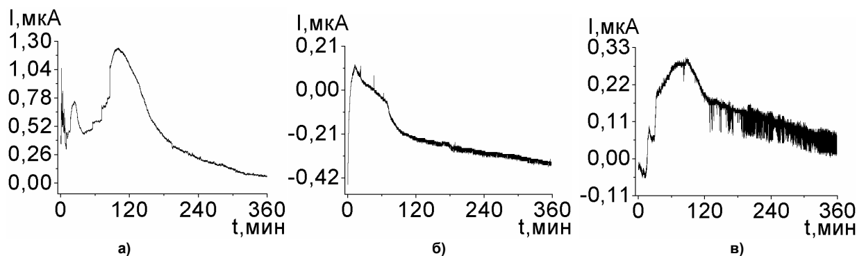
Рис. 1. Изменение тока поляризации гелей ГОЦ, магнитное поле отсутствует; три параллельных образца синтезировали при \text{pH} = 9,25 ; длина электрохимической ячейки L = 7 см; количество ГОЦ в ячейке n = 0,00094 моль
